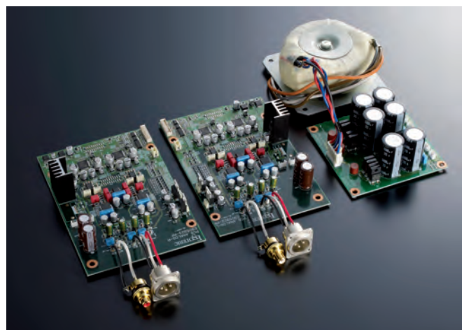
Le sezioni analogiche di uscita, i due circuiti RCA/XLR, la parte di filtraggio e stabilizzazione e il trasformatore dedicato.
